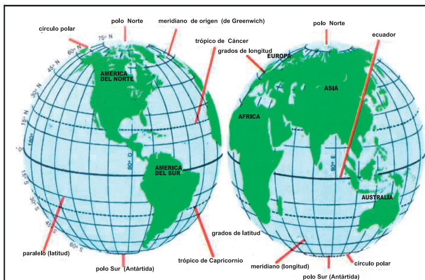
Paralelos y meridianos de la Tierra
