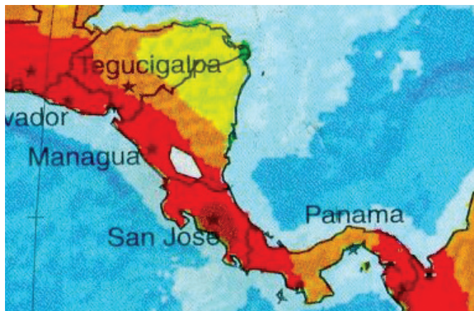
Áreas vulnerables Sísmica
