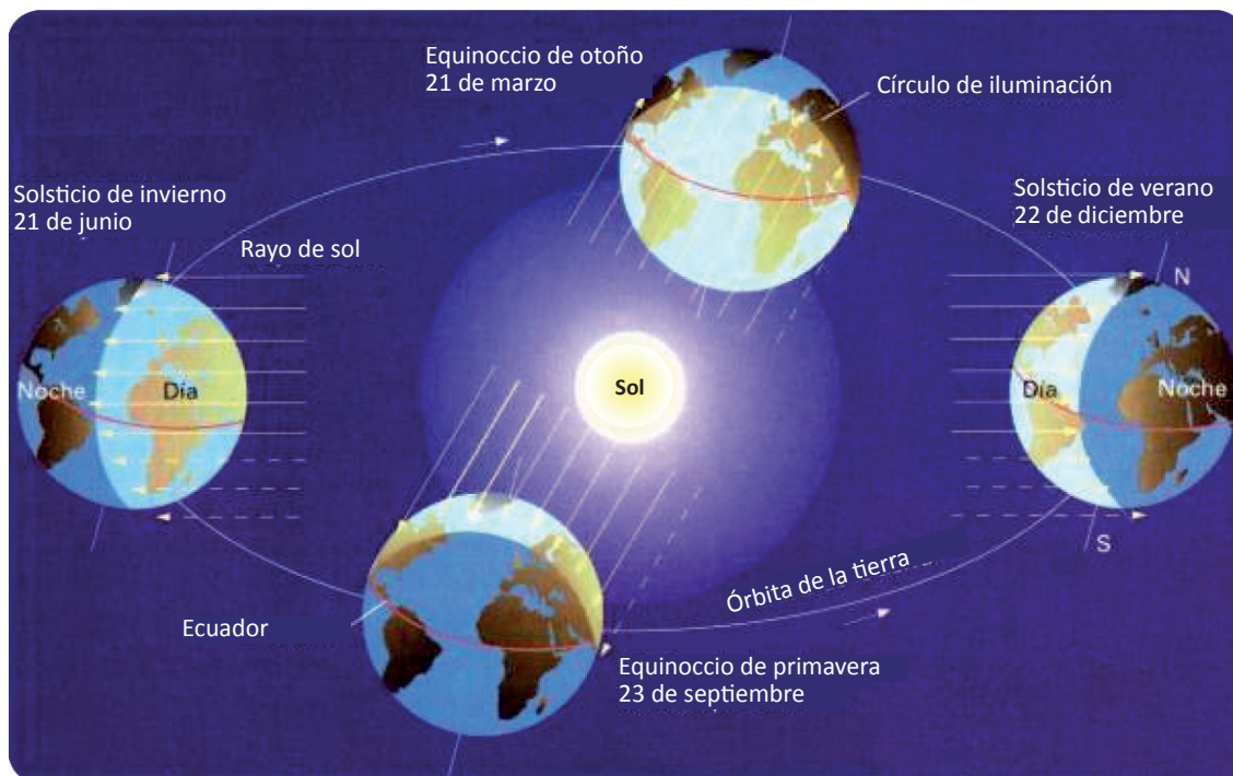
Estaciones del año
