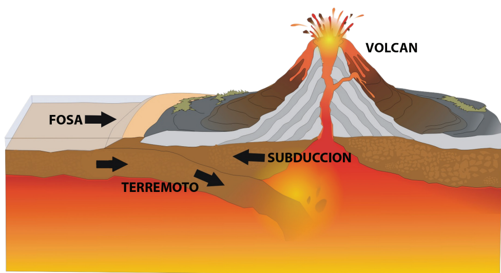
Choque de las placas
