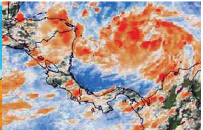
Áreas vulnerables a Huracanes
