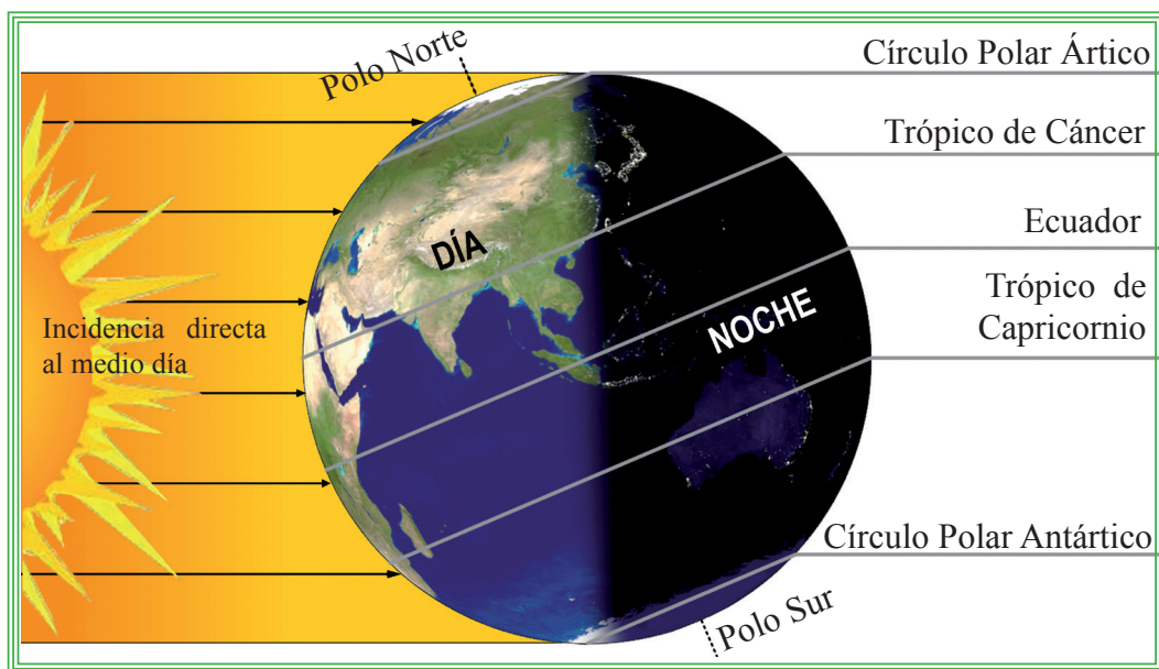
El Sol iluminando una parte de la Tierra
