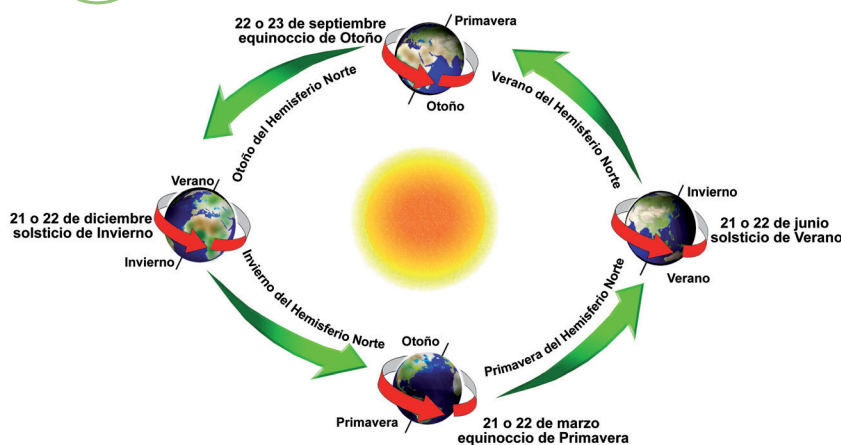
Movimiento de traslación
