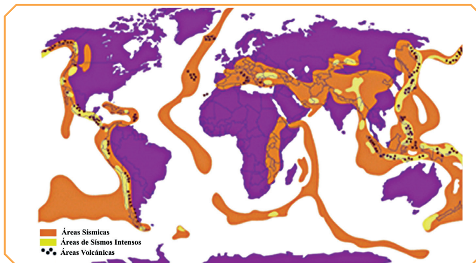
Mapa de las principales Zonas Sísmicas y Volcánicas
