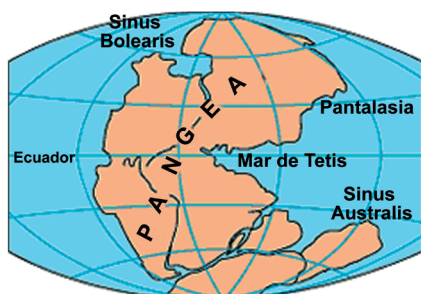
200 millones de años atrás
