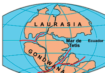
Hace 180 millones de años
